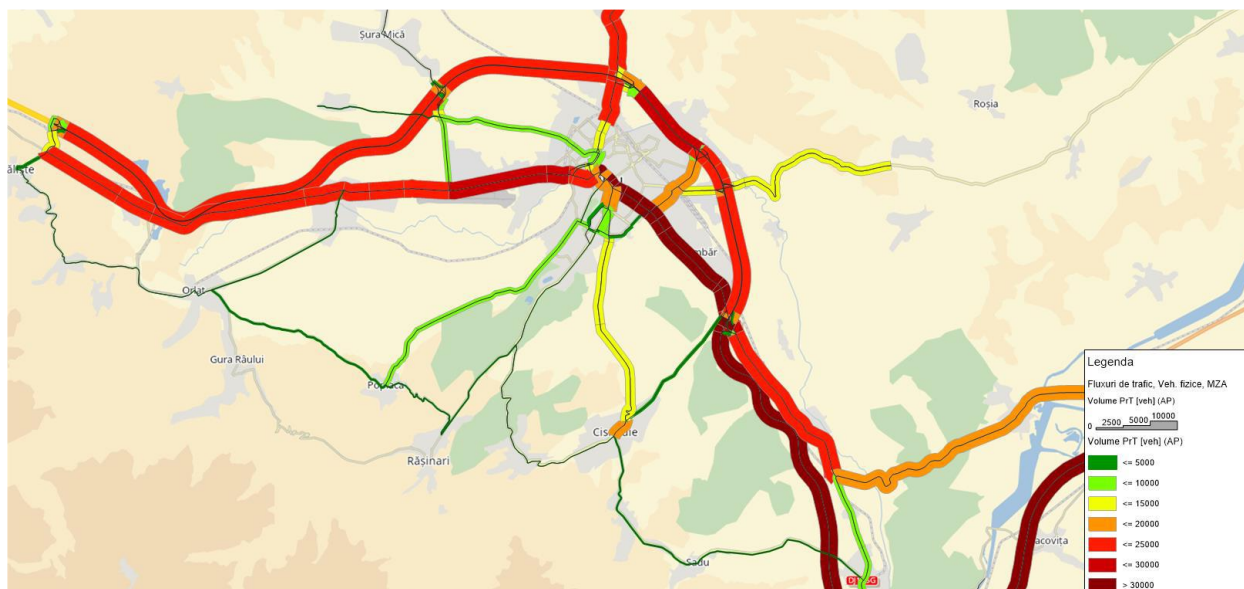
Figura nr. 13 Fluxuri de trafic - Scenariul de referinta – 2050
