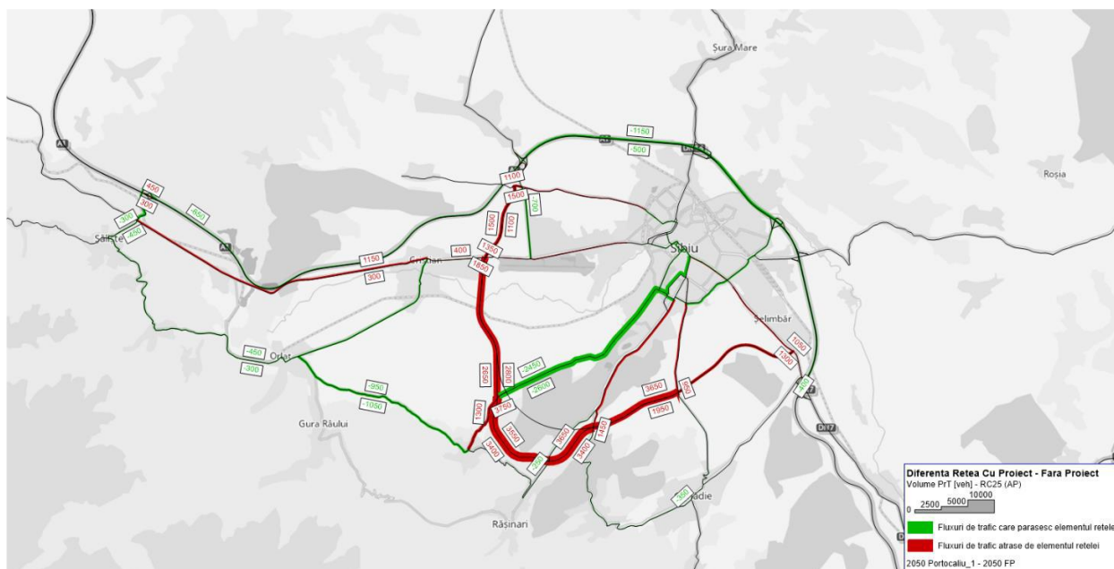
Figura nr. 15 Redistribuirea fluxurilor de trafic în scenariul cu proiect - Scenariul de referință – 2025
