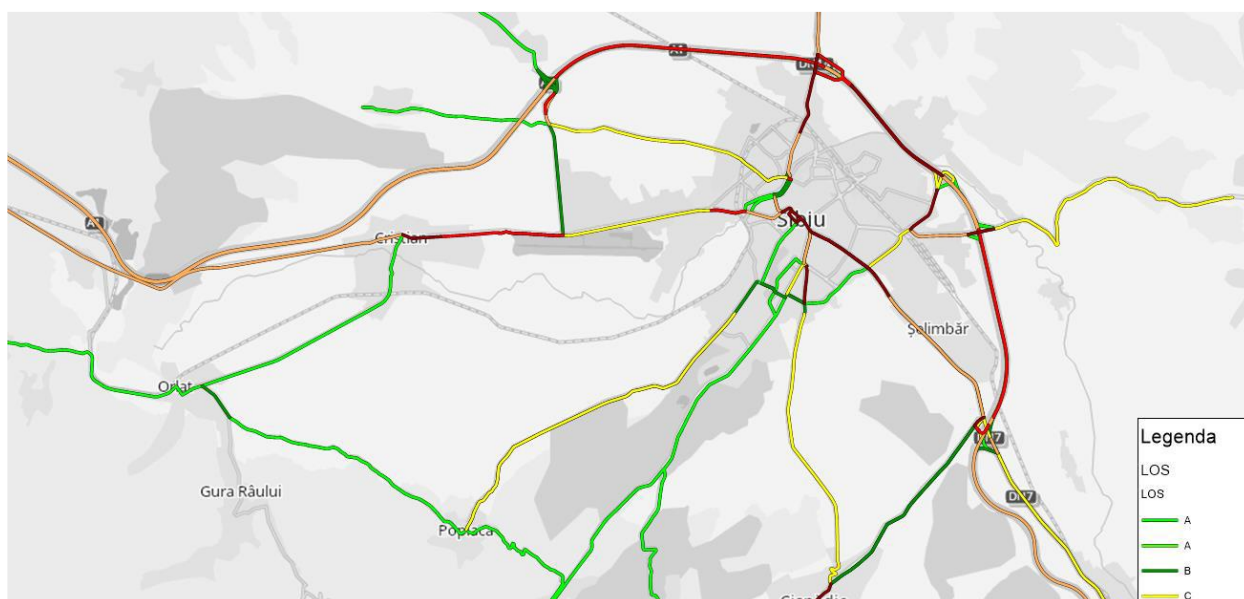
Figura nr. 23 Raportul volum/capacitate (nivel de serviciu) – scenariul fără proiect-2050
