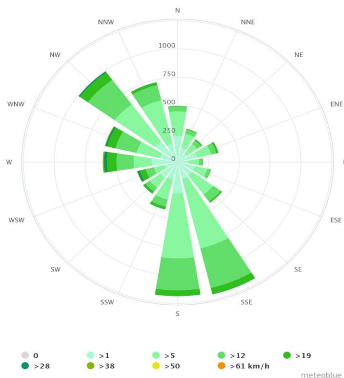
Figura nr. 32 Direcția predominantă a vânturilor (sursa : meteoblue)
