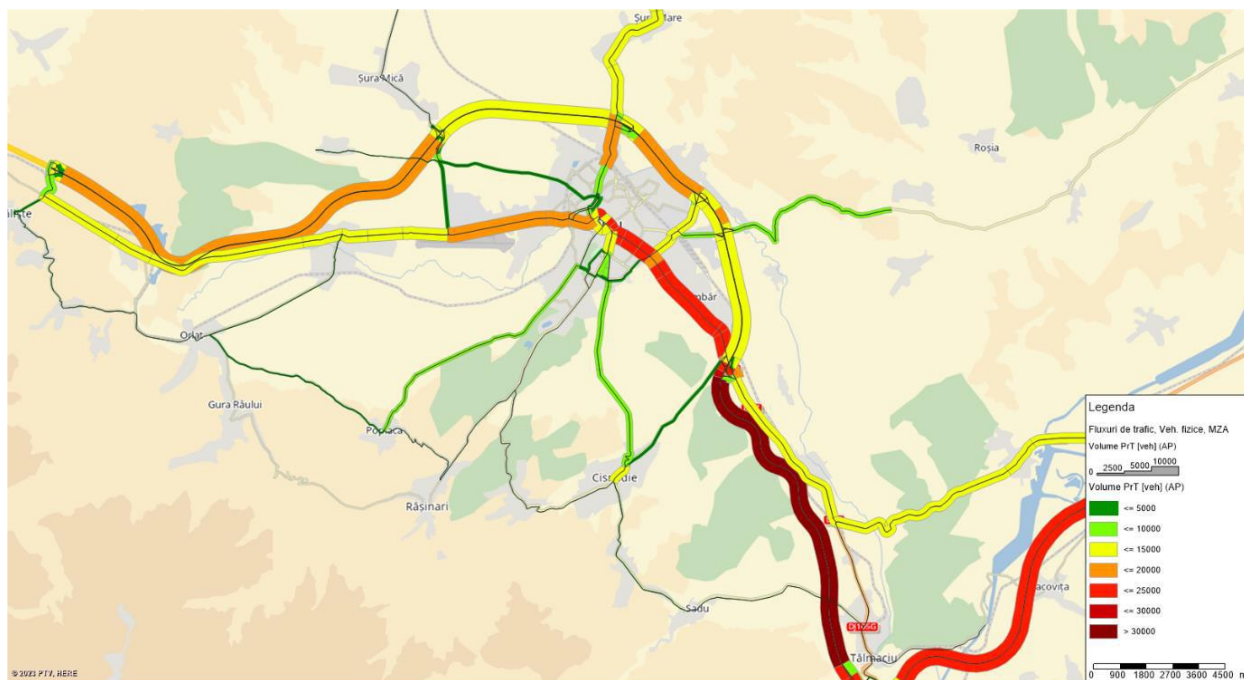
Figura nr. 10 Fluxuri de trafic - Scenariul de referinta – 2025
