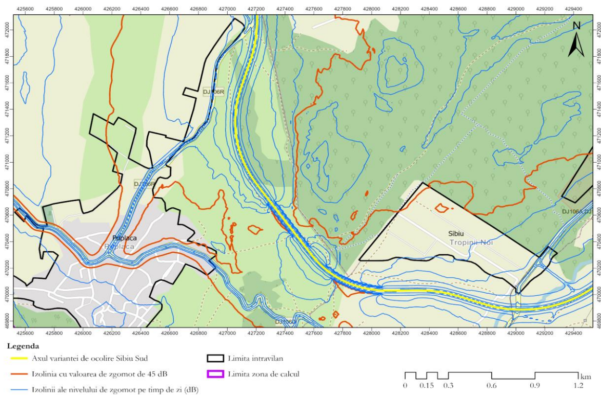
Figura nr. 47 Rezultatele modelării de zgomot pe timp de noapte în etapa de operare – Poblaca
