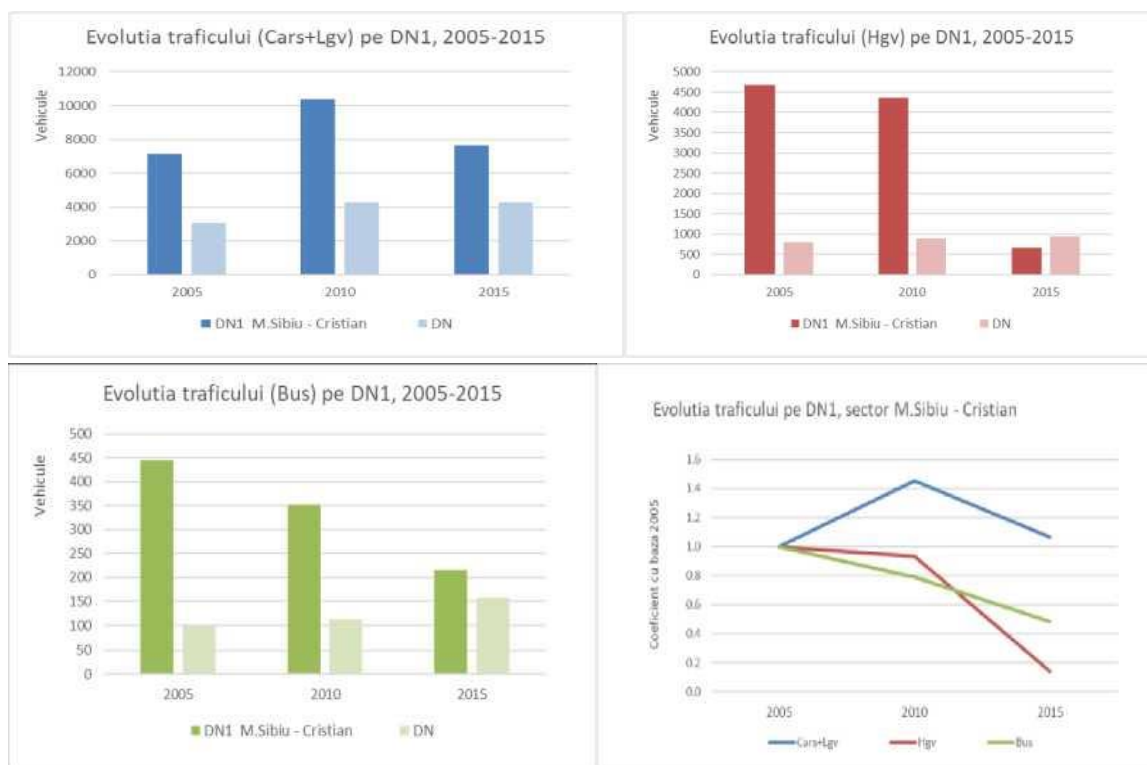
Figura nr. 7 Evolutia traficului pe categorii de vehicule, DN1, sector omogen M.Sibiu - Cristian (Sursa: Studiu de trafic - CESTRIN, Recensamantul general de circulatie 2005, 2010, 2015)
