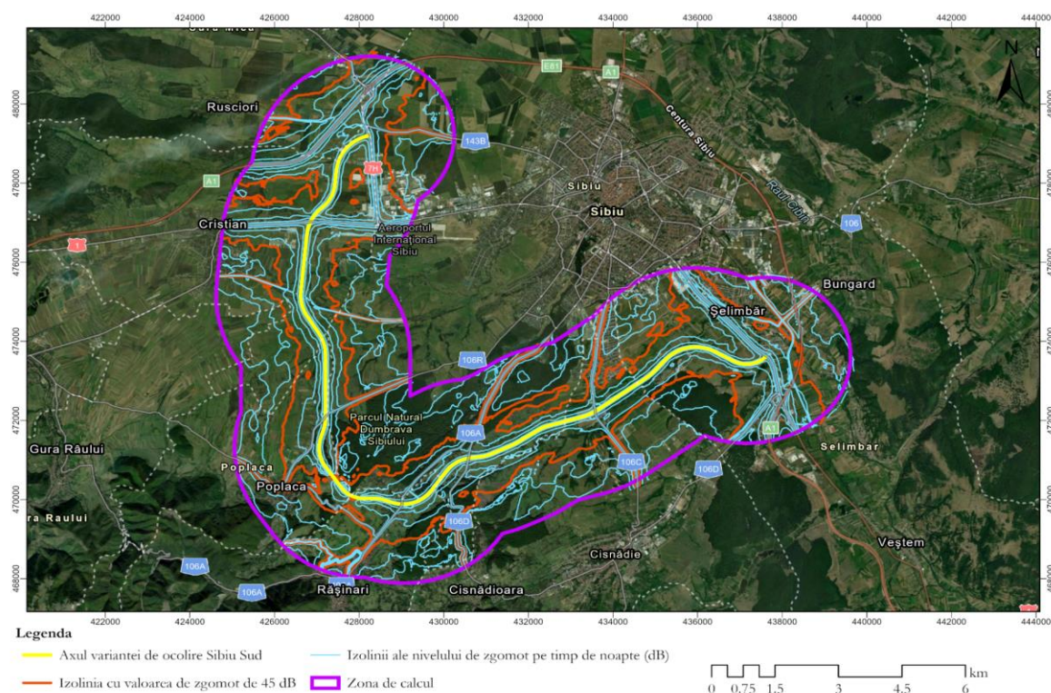
Figura nr. 45 Rezultatele modelării de zgomot pe timp de noapte în etapa de operare – scenariul anului 2050 (impact cumulativ cu traficul existent din zona de studiu)
