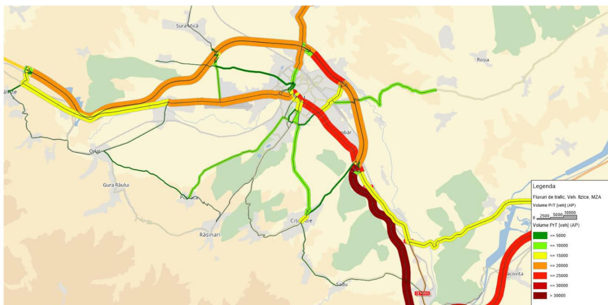
Figura nr. 11 Fluxuri de trafic - Scenariul de referinta – 2030
