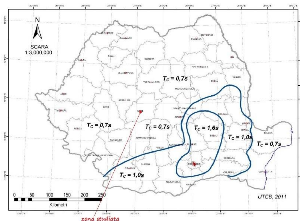
Zonarea teritoriala a Romaniei in termeni de perioada de control (colt), T_c a spectrului de raspuns
